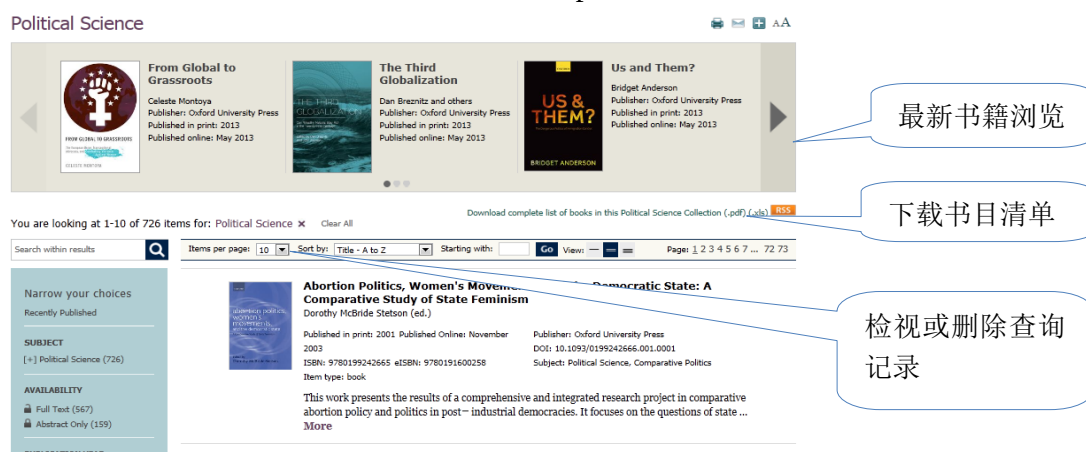
图 3 学科页面
