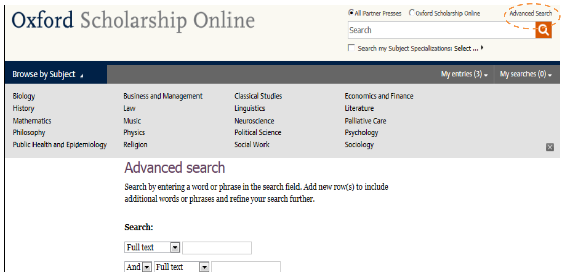
图6 高级检索
